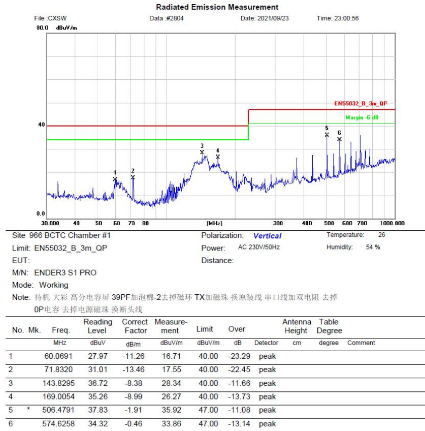
图 4-6 辐射测试垂直方向
