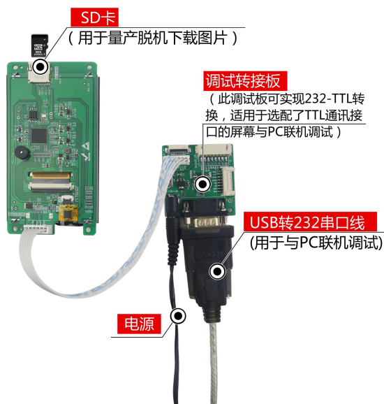
图 1-5 调试工具图
