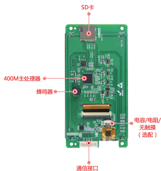
图 1-4 硬件配置图
