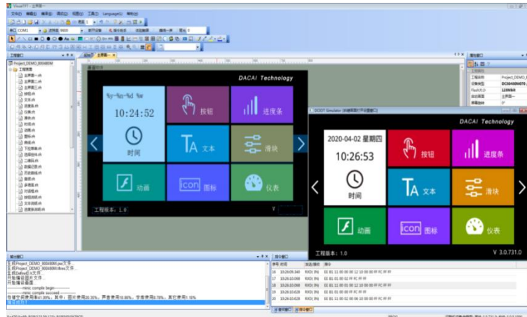
图 9-1 VisualTFT 主界面
